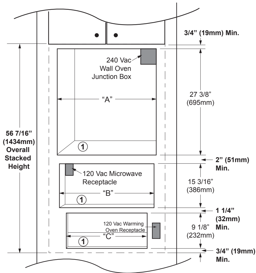
CUTOUT DIMENSIONS
