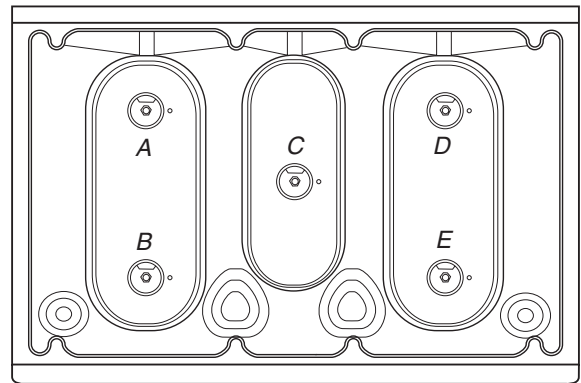
A. Brûleur standard - gicleur pour gaz propane numéro 78 B. Brûleur haute puissance - gicleur pour gaz propane numéro 80 C. Brûleur central - gicleur pour gaz propane numéro 80 D. Brûleur standard - gicleur pour gaz propane numéro 78 E. Brûleur standard - gicleur pour gaz propane numéro 78
