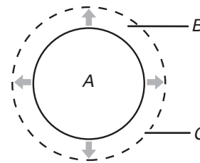
A. Área de cocción en la superficie B. Utensilio de cocina/ensavador C. 1/2" (1,3 cm) de saliente máxima
