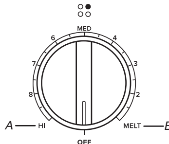
A. Opción de calor Hi (Alto) B. Opción Melt (Derretir)
